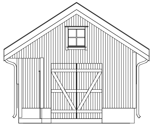
Fasade - Sør 1 : 100
