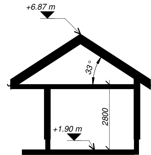
Snitt A-A 1 : 100
