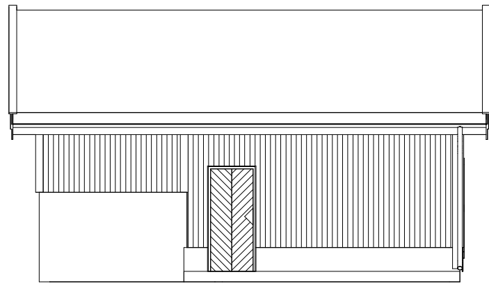
Fasade - Vest 1 : 100
