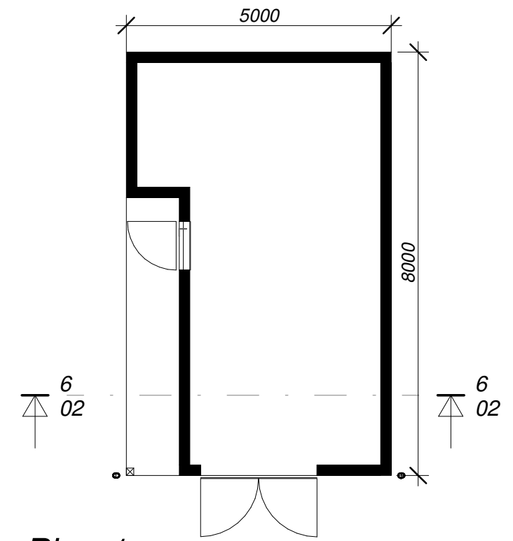
Plan 1 1 : 100
