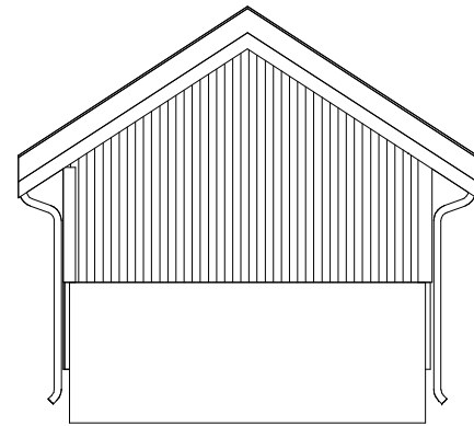
Fasade - Sør 1 : 100
