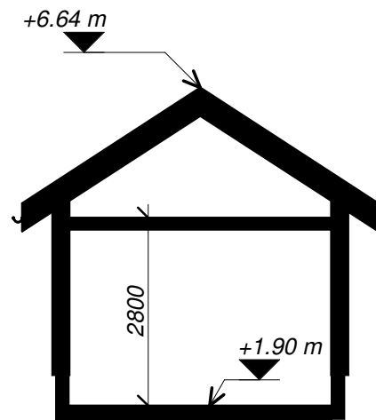
Snitt A-A 1 : 100
